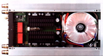
L'intérieur bien rempli du Primo Cento VT ou la sophistication pacifique pour le musicien. En haut à gauche, l'ajustage phono utilisant des amplificateurs opérationnels.
