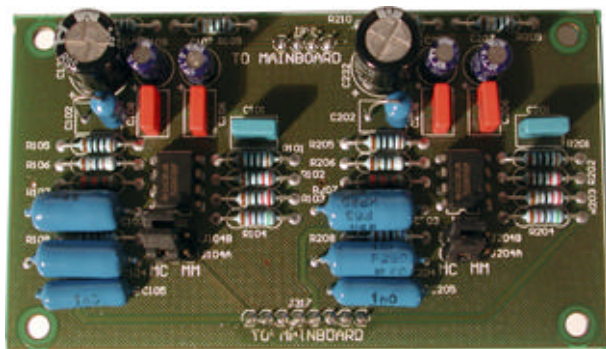
Module d'entrée Phono (en option)
